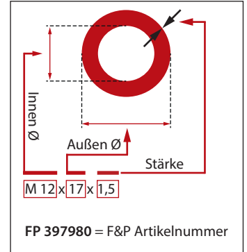
Dichtring / gasket
